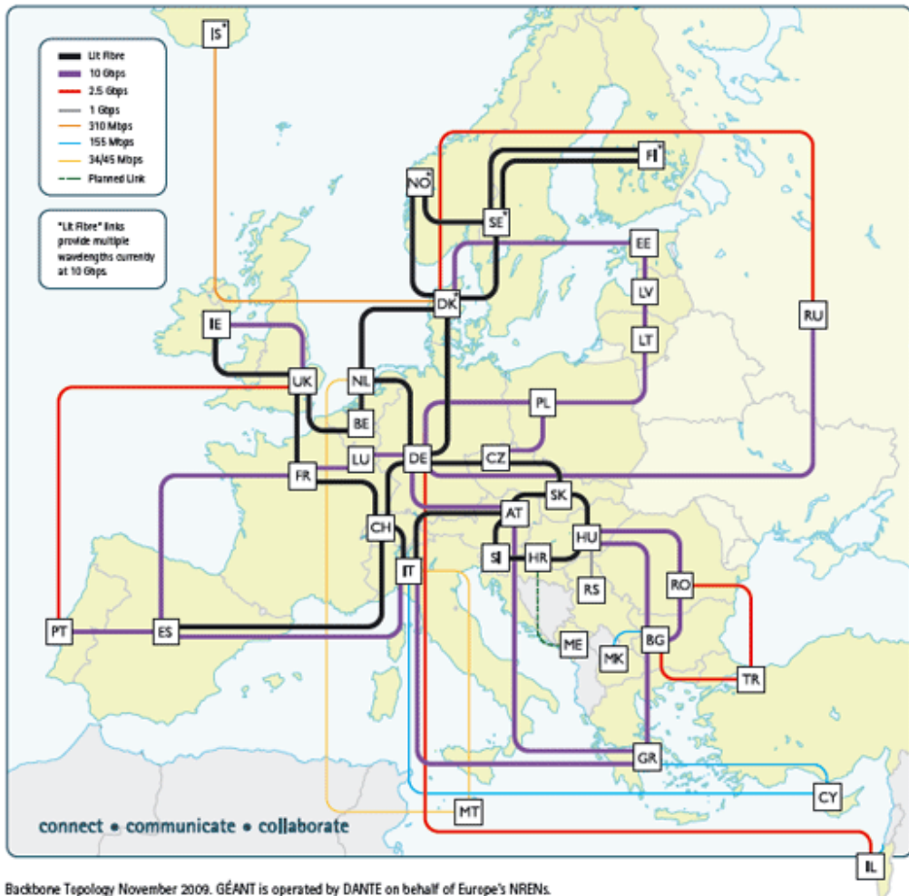
Figura 1: Topología de la troncal de GÉANT, noviembre de 2009 (ver original en: http://www.geant.net/Network/NetworkTopology/pages/home.aspx ).
